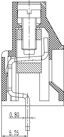
SECTION A-A
